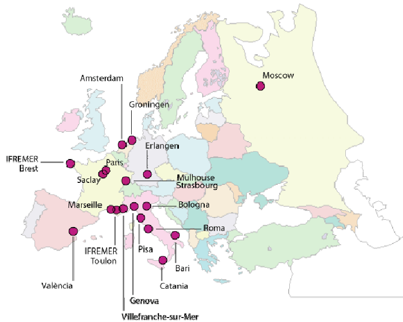
Figure B-10 : Carte des laboratoires participants à la construction du télescope Antares.
