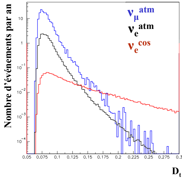
Figure D-19 : Distributions de la densité temporelle des coups des événements reconstruits, les \nu_\mu^{atm} en bleu, les \nu_e^{atm} en noir et les \nu_e^{cos} en rouge, en échelle logarithmique.
