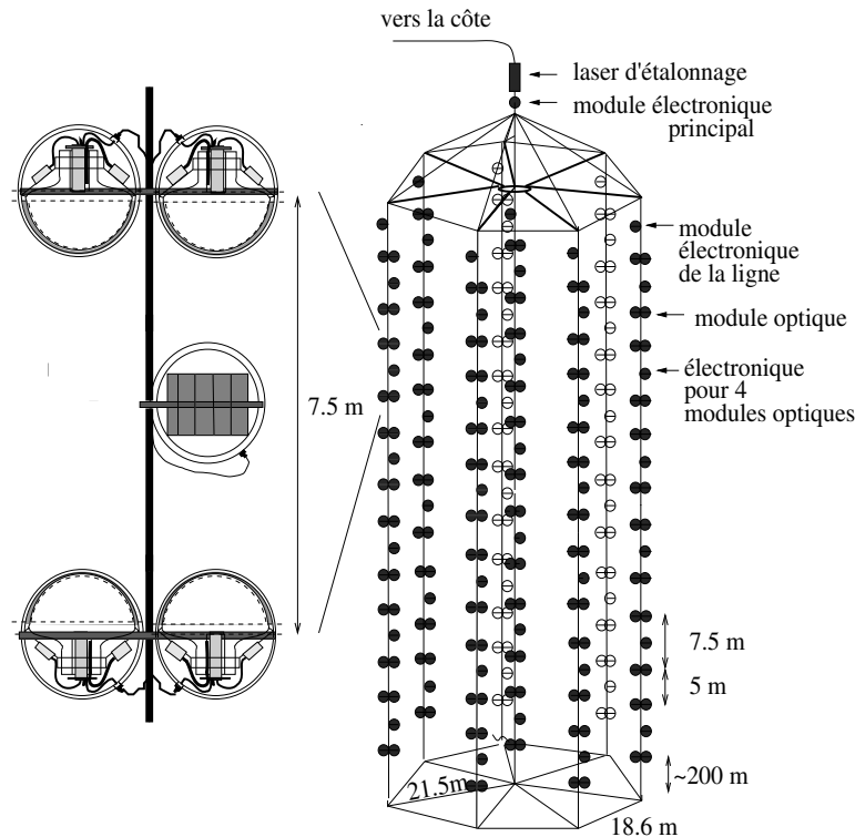
Figure B-31 : Schéma du détecteur Baïkal NT200.
