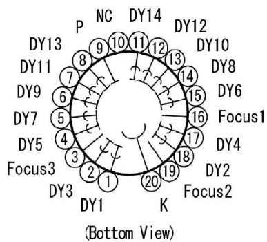
FIG. 5.21 – Le PM 10" R7081-20 d'Hamamatsu, utilisé par ANTARES
